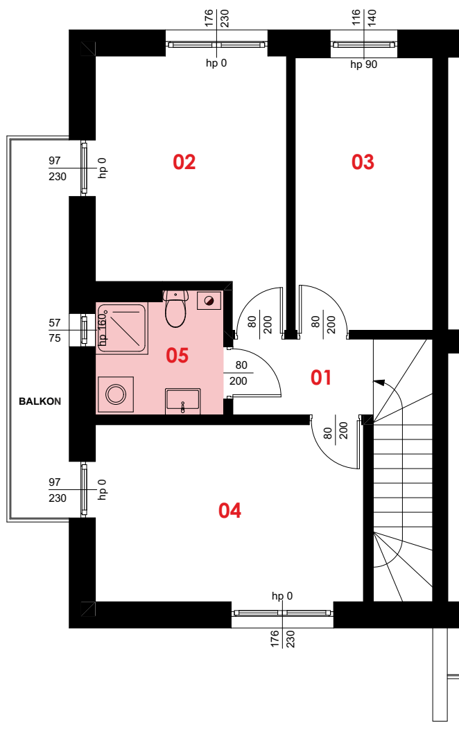
RZUT I PIĘTRA
