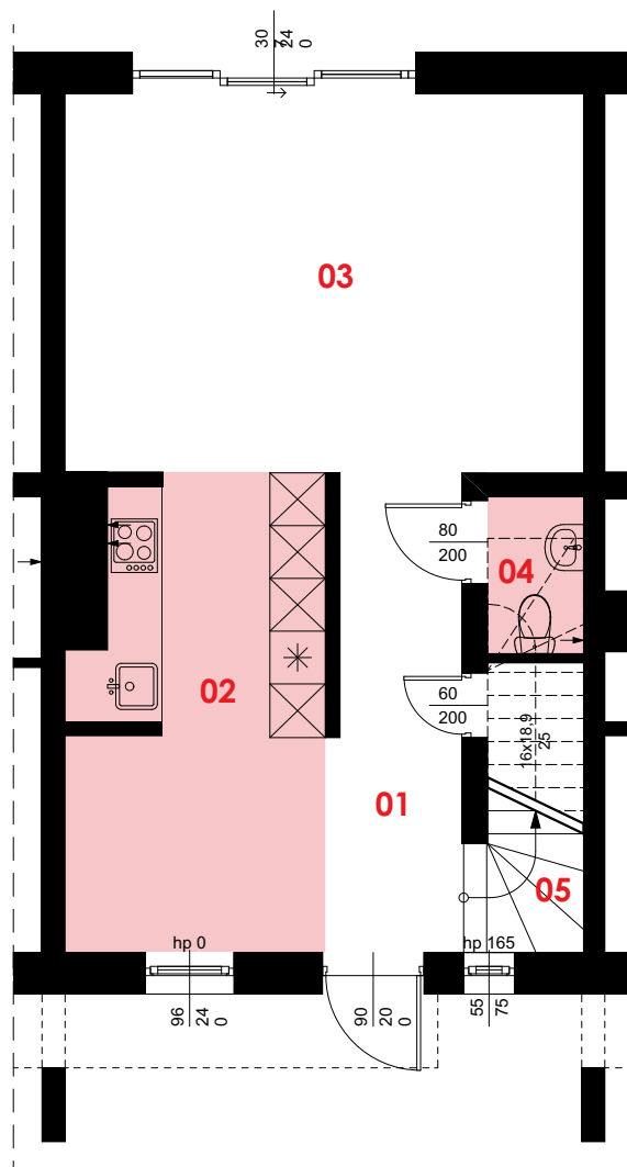
RZUT PRZYZIEMIA
