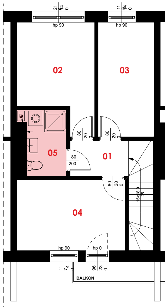
RZUT I PIĘTRA
